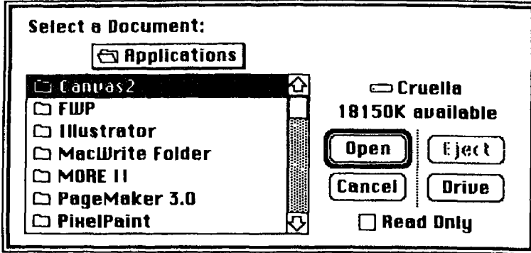
شكل (٩-٥) : صندوق حوار نمطى لخير GetFile .
